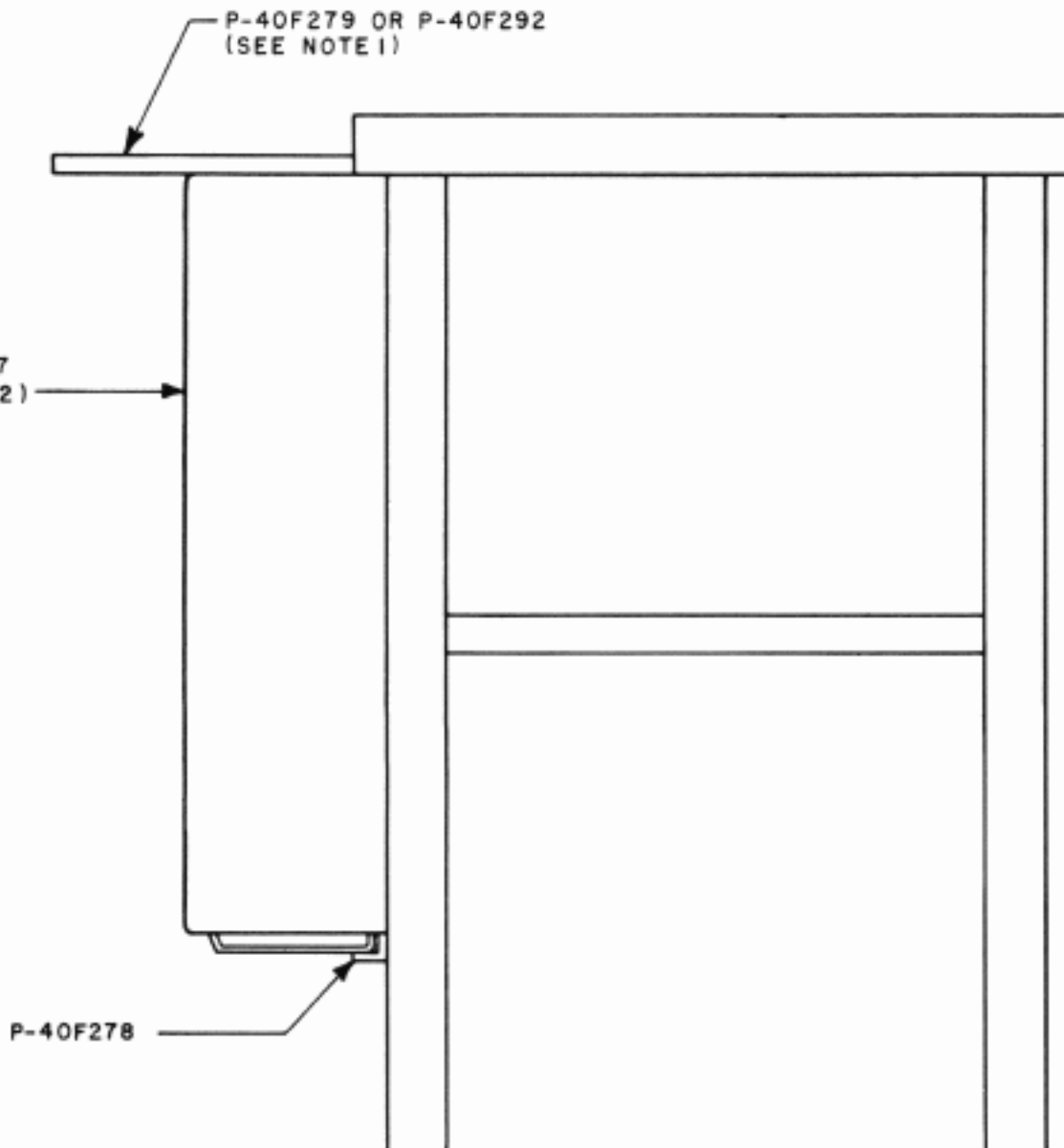
FRONT VIEW (SUBSET NOT SHOWN)
