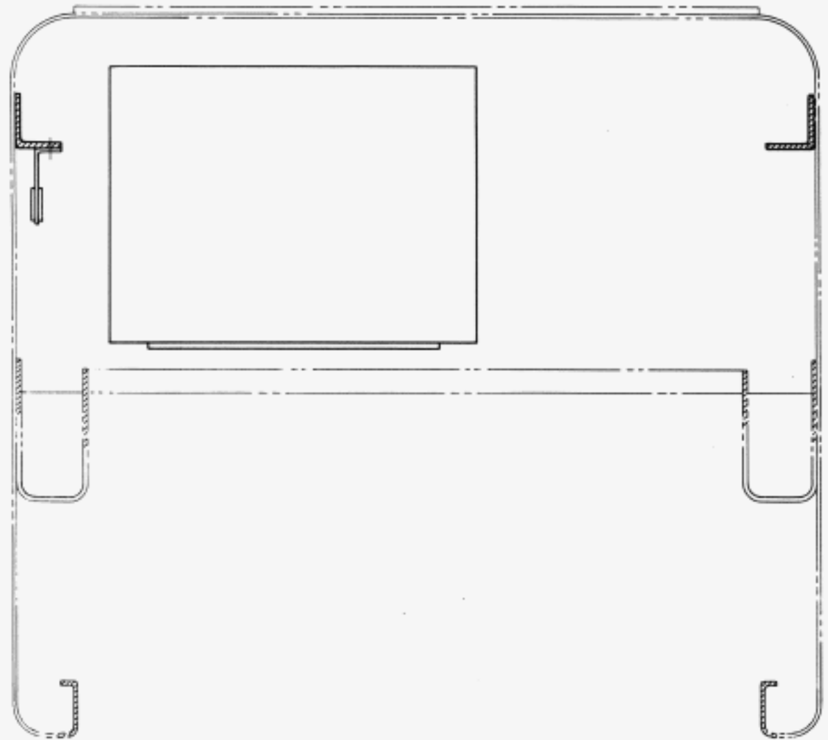
SECT A-A
