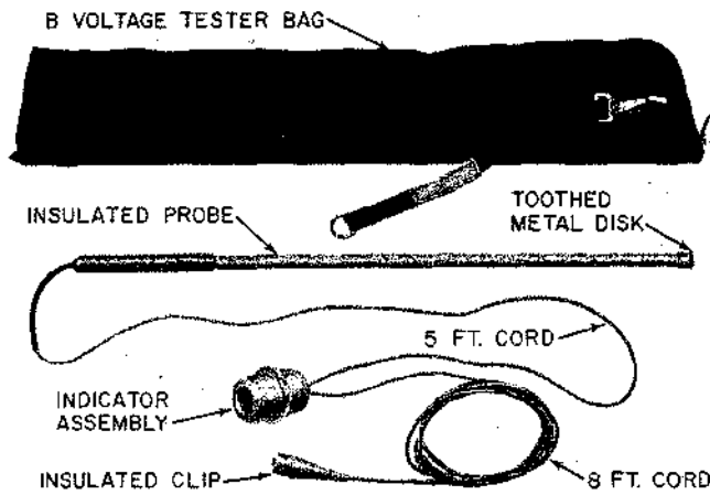
Fig. 1—B-Voltage Tester
