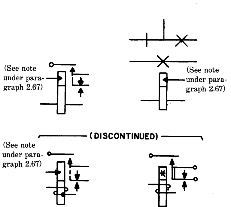
(d) Relay with preliminary make-contact
