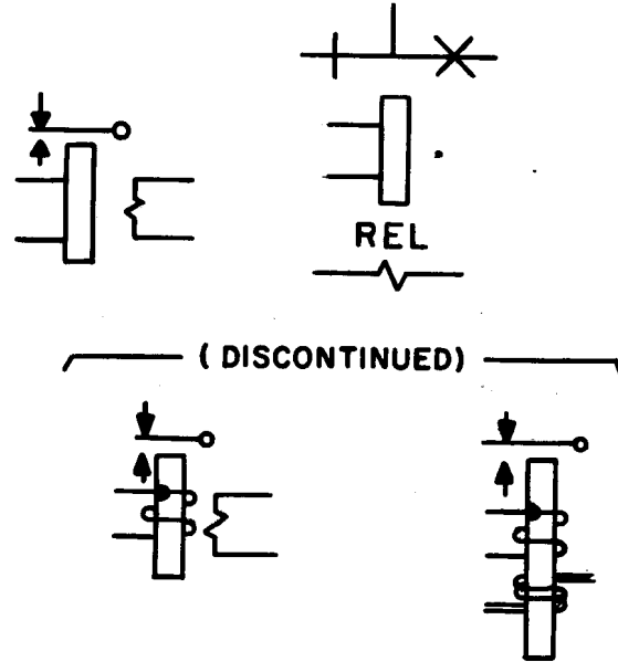
(d) Relay with preliminary make-contact
