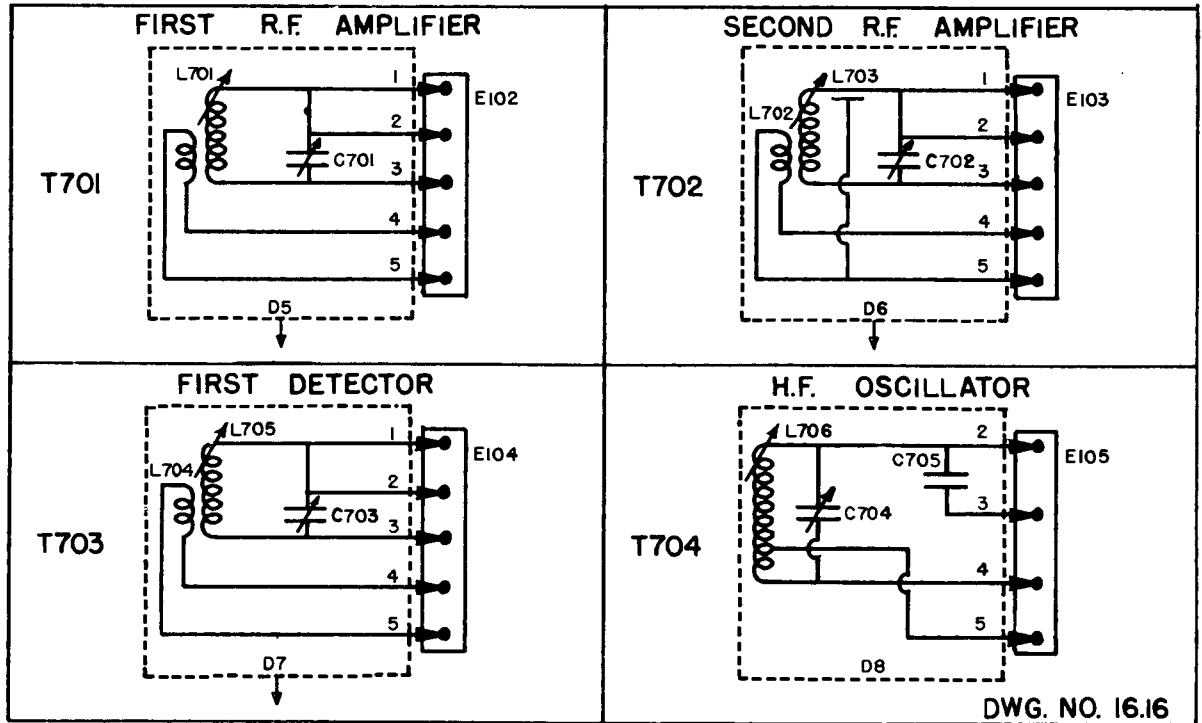
ACTUAL WIRING DIAGRAM TYPE CNA-47159 COIL SET 4
