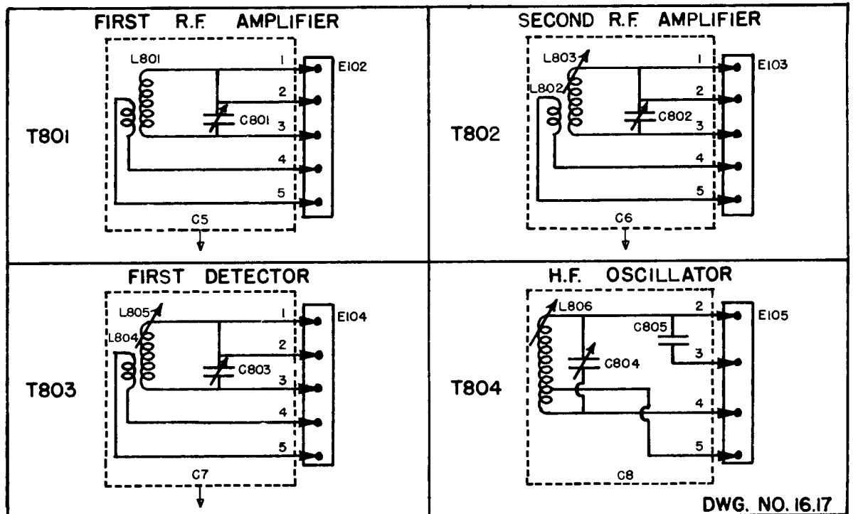
ACTUAL WIRING DIAGRAM TYPE CNA-47160 COIL SET 5
