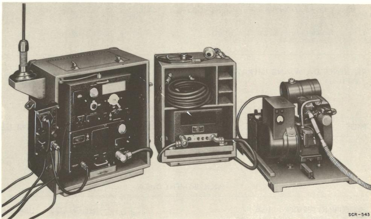
SCR-543
